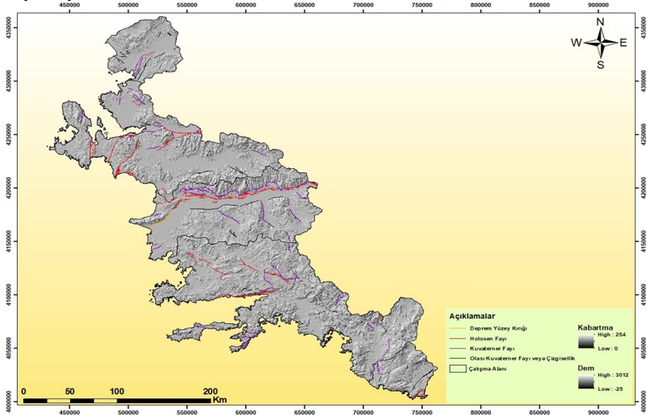
Şekil 3. Çalışma alanı diri fay haritası
